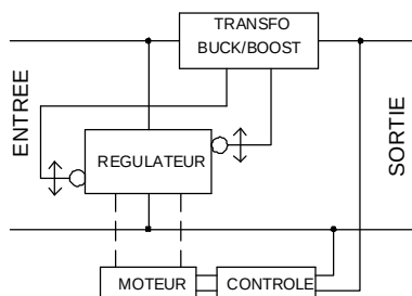
chaîne de régulation monophasée
