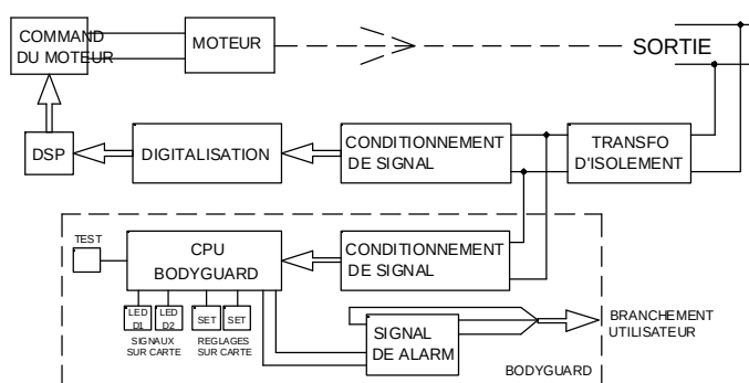
solution avec microprocesseur de supervision
